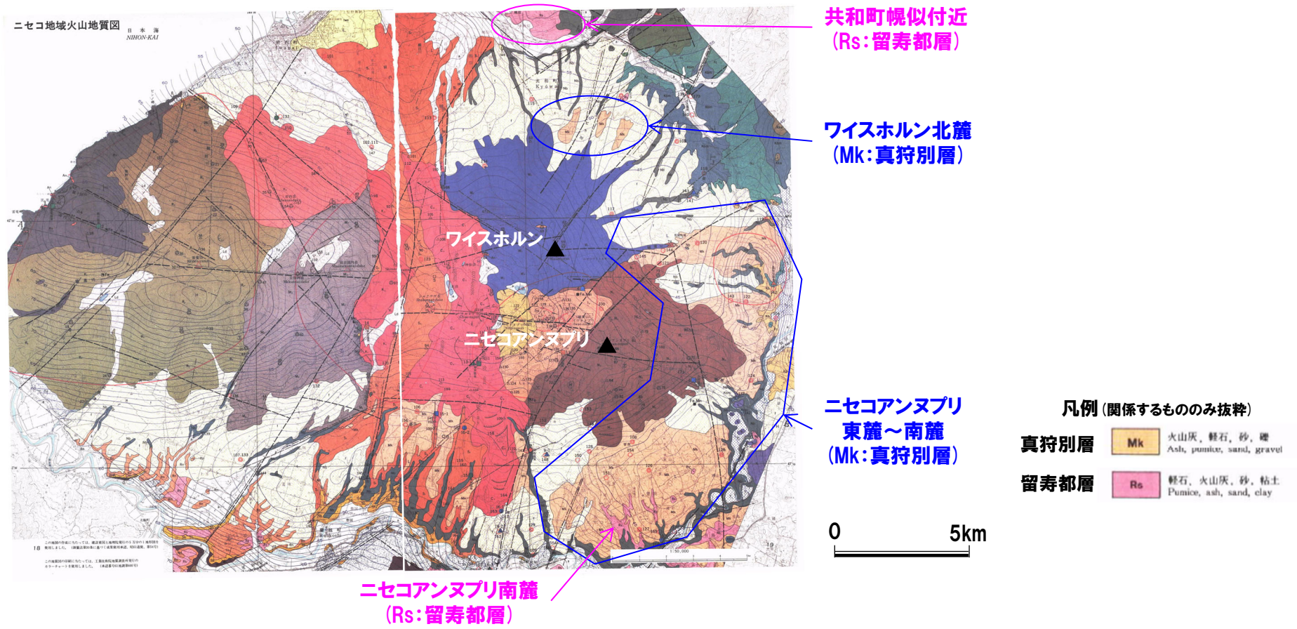
ニセコ地域火山地質図 (新エネルギー総合開発機構 (1987a) に加筆)
