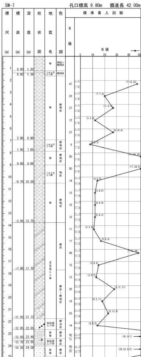
添付 1-37 図(1/2) ボーリング柱状図・コア写真 (SW-7)
