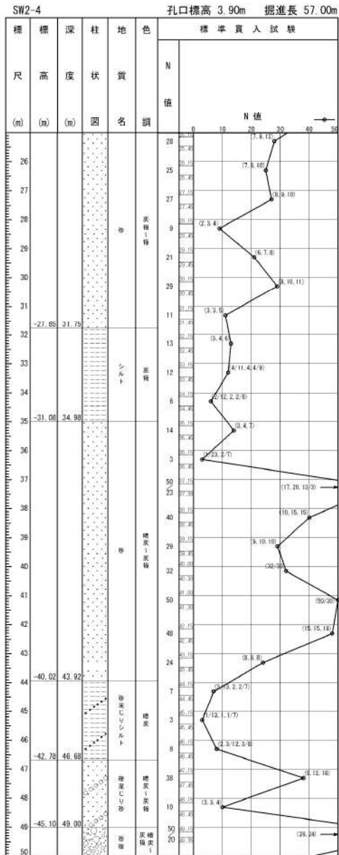
添付 1-2 図(2/3) ボーリング柱状図・コア写真 (SW2-4)
