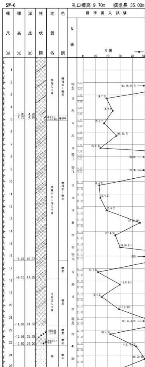
添付 1-36 図(1/2) ボーリング柱状図・コア写真 (SW-6)
