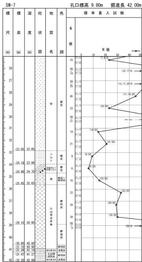
添付 1-37 図(2/2) ボーリング柱状図・コア写真 (SW-7)
