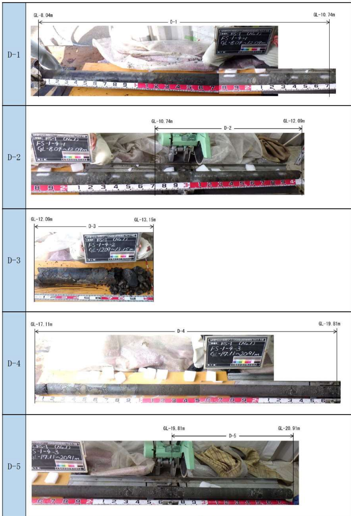
添付 1-24 図(9/10) ボーリング柱状図・コア写真 (FS-1)
