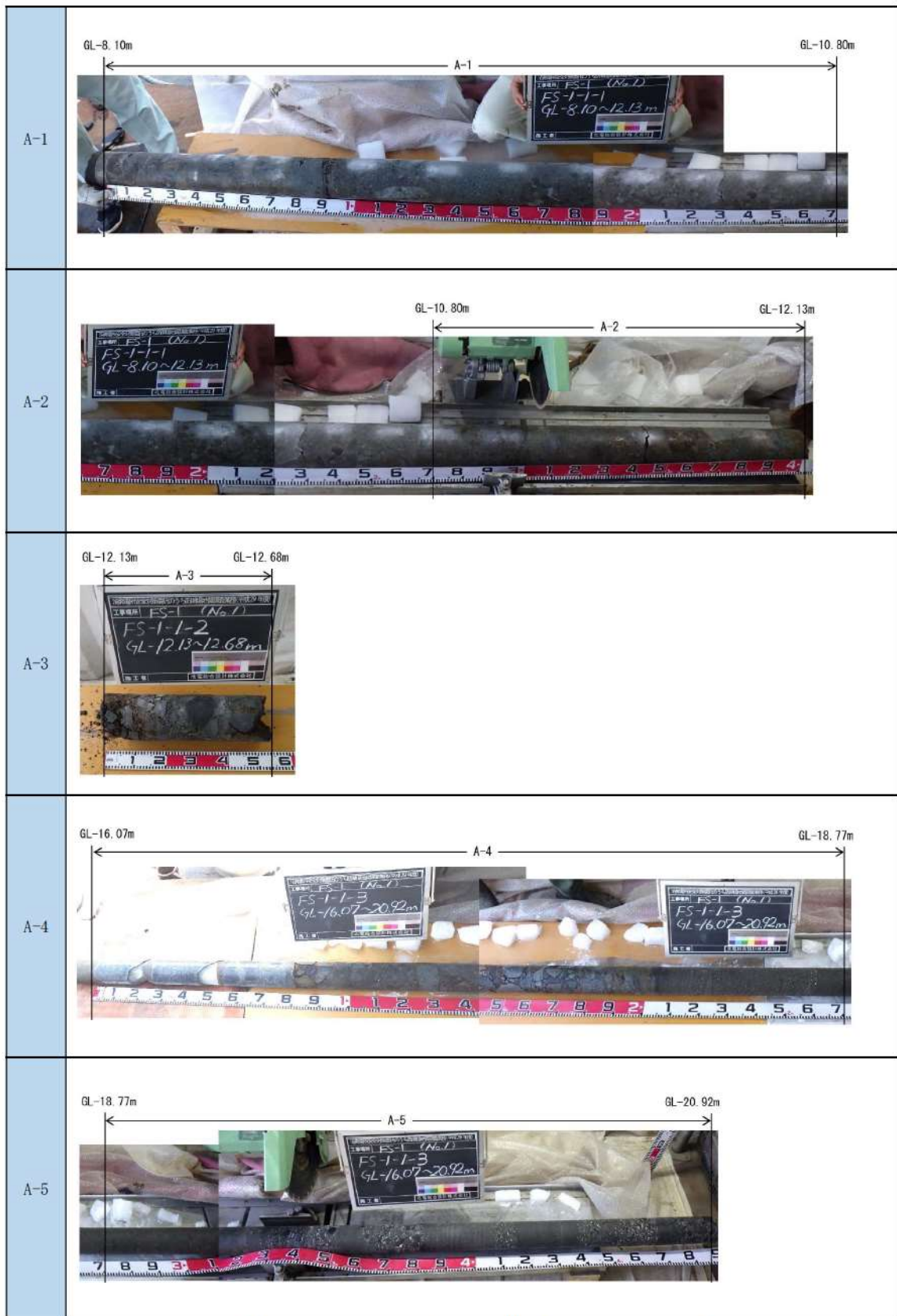
添付 1-24 図(3/10) ボーリング柱状図・コア写真 (FS-1)
