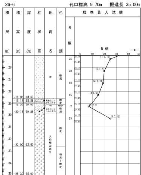
添付 1-36 図(2/2) ボーリング柱状図・コア写真 (SW-6)
