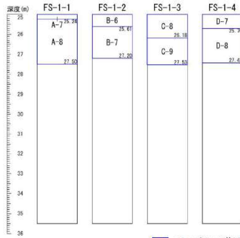
添付 1-24 図(2/10) ボーリング柱状図・コア写真 (FS-1)
