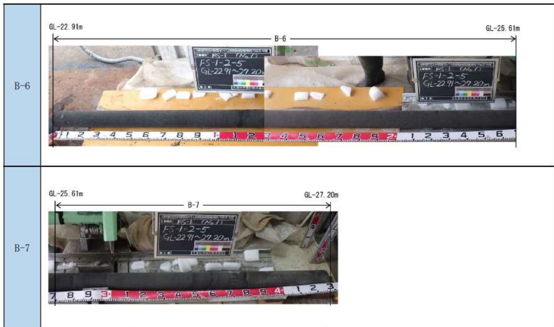
添付 1-24 図(6/10) ボーリング柱状図・コア写真 (FS-1)
