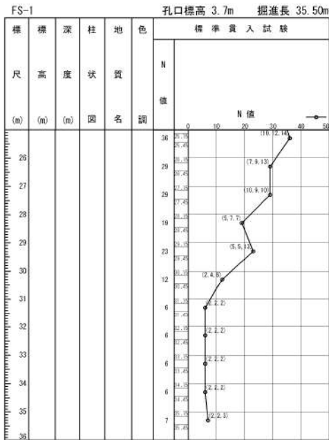
添付 1-24 図(2/10) ボーリング柱状図・コア写真 (FS-1)
