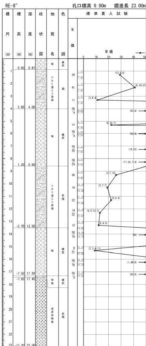
添付 1-30 図 ボーリング柱状図・コア写真 (RE-8" )
