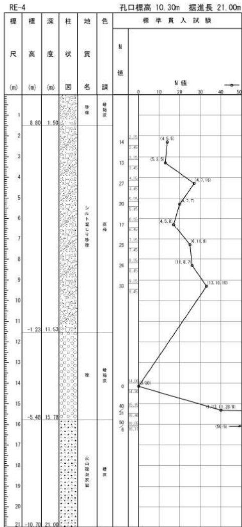
添付 1-7 図 ボーリング柱状図・コア写真 (RE-4)
