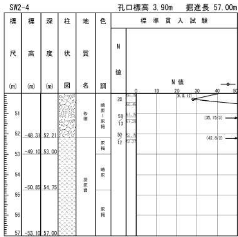
添付 1-2 図(3/3) ボーリング柱状図・コア写真 (SW2-4)
