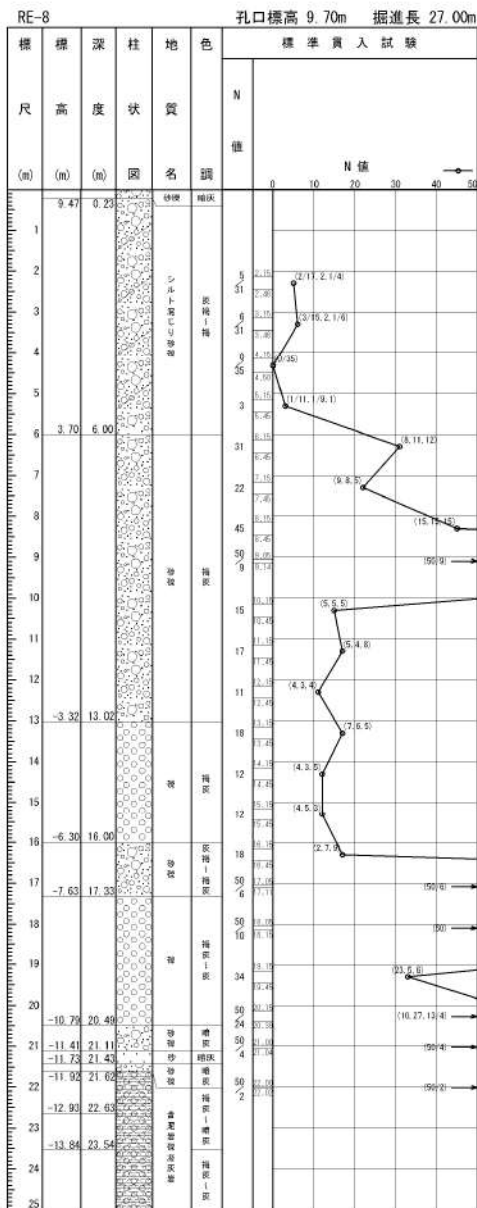
添付 1-29 図(1/2) ボーリング柱状図・コア写真 (RE-8)
