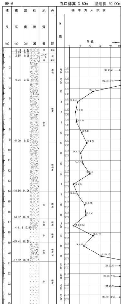
添付 1-9 図(1/3) ボーリング柱状図・コア写真 (RE-6)
