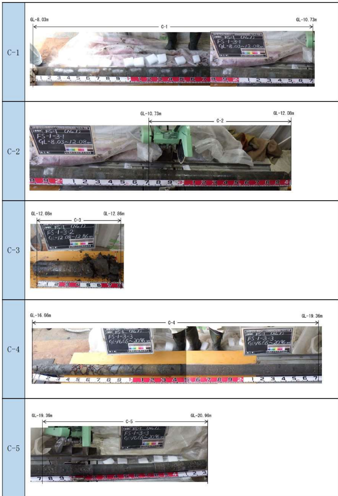
添付 1-39 図(7/10) ボーリング柱状図・コア写真 (FS-1)
