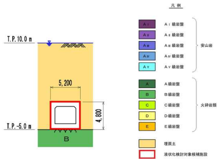
第 3.2-12 図 原子炉補機冷却海水管ダクト断面図
