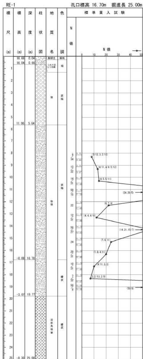
添付 1-4 図 ボーリング柱状図・コア写真 (RE-1)
