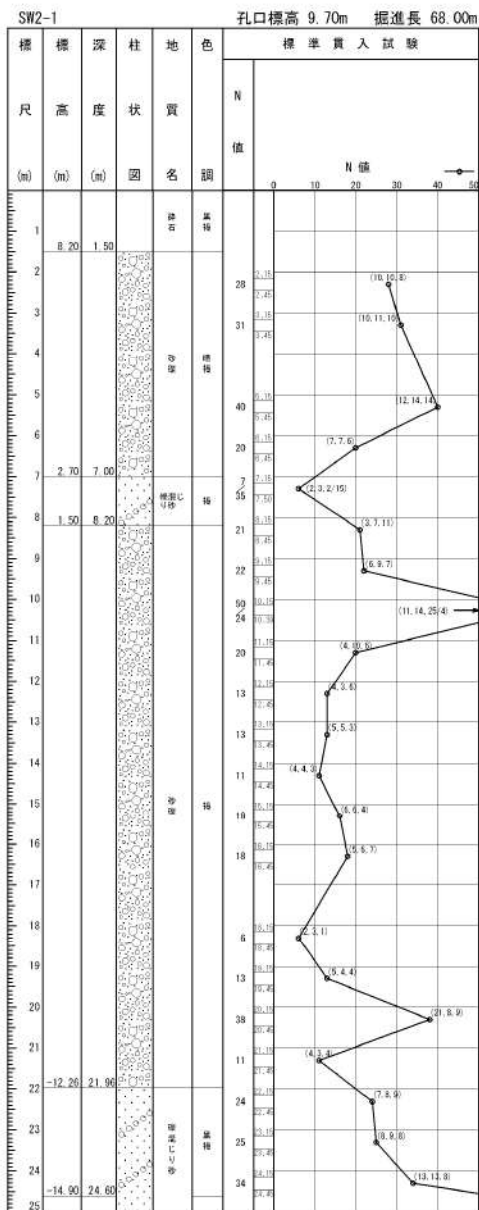
添付 1-25 図(1/3) ボーリング柱状図・コア写真 (SW2-1)
