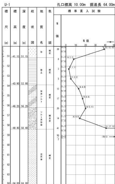
添付 1-32 図(3/3) ボーリング柱状図・コア写真 (U-1)
