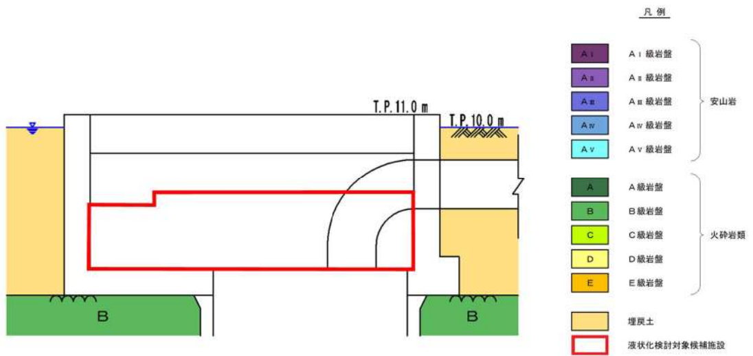
第 3.2-16 図 3号炉放水ピット流路縮小工断面図
