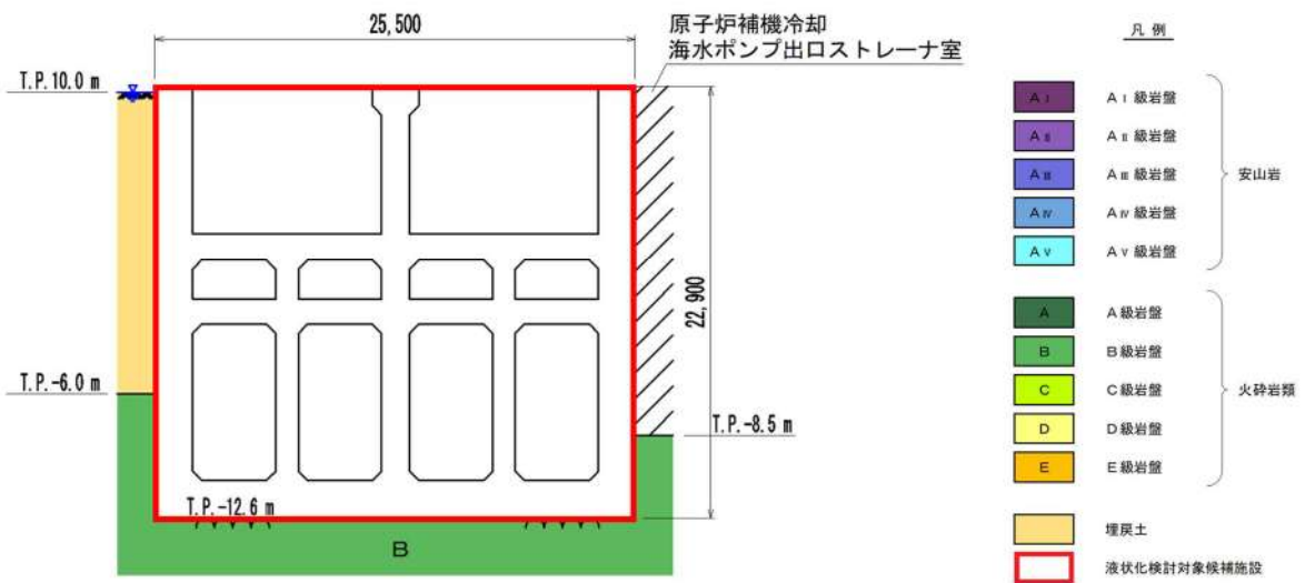
第 3.2-10 図 取水ピットポンプ室断面図
