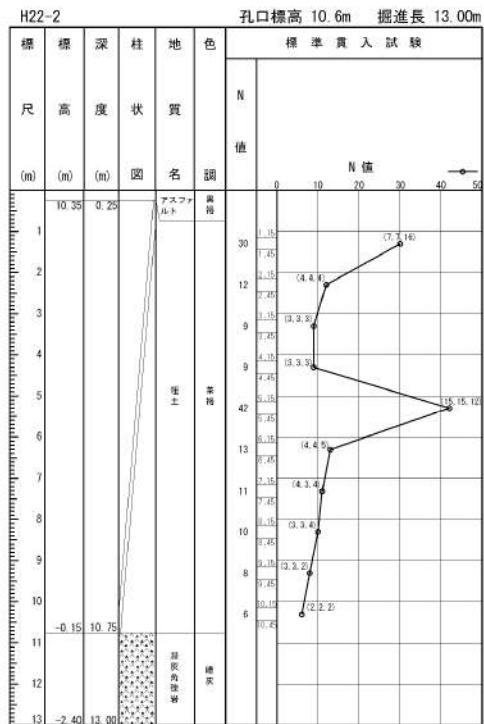
添付 1-19 図 ボーリング柱状図・コア写真 (H22-2)
