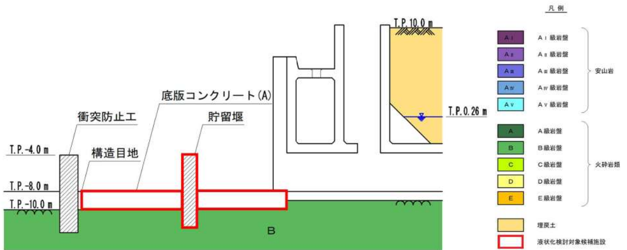
第 3.2-20 図 貯留堰部断面図
