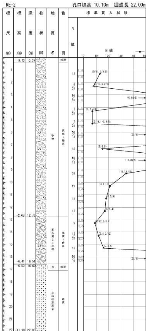
添付 1-5 図 ボーリング柱状図・コア写真 (RE-2)
