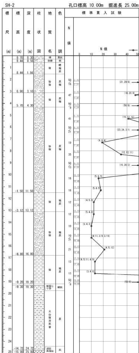
添付 1-31 図 ボーリング柱状図・コア写真 (SH-2)
