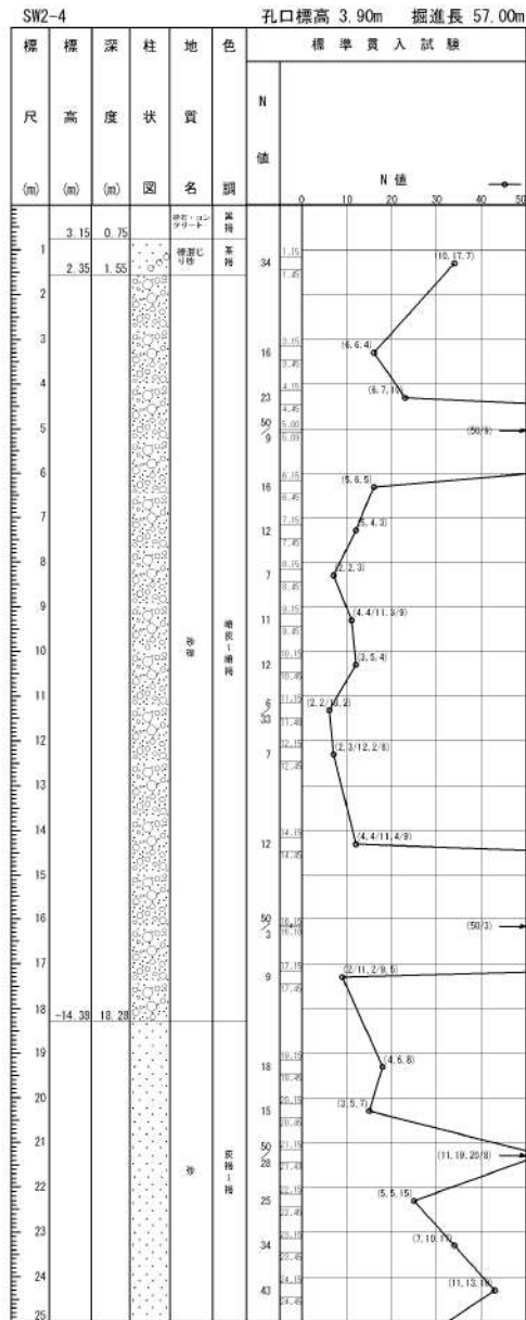
添付 1-2 図(1/3) ボーリング柱状図・コア写真 (SW2-4)
