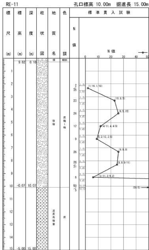
添付 1-23 図 ボーリング柱状図・コア写真 (RE-11)
