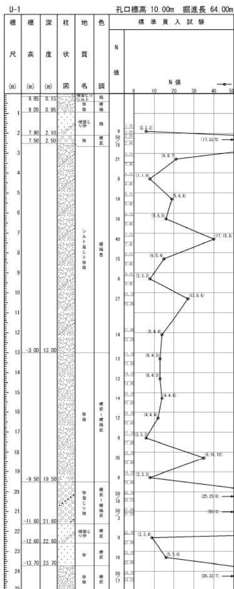
添付 1-32 図(1/3) ボーリング柱状図・コア写真 (U-1)
