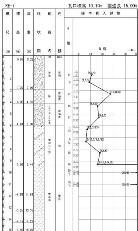
添付 1-28 図 ボーリング柱状図・コア写真 (RE-7)
