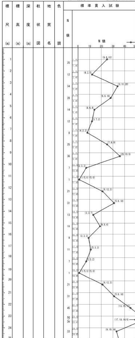
添付 1-24 図(1/10) ボーリング柱状図・コア写真 (FS-1)
