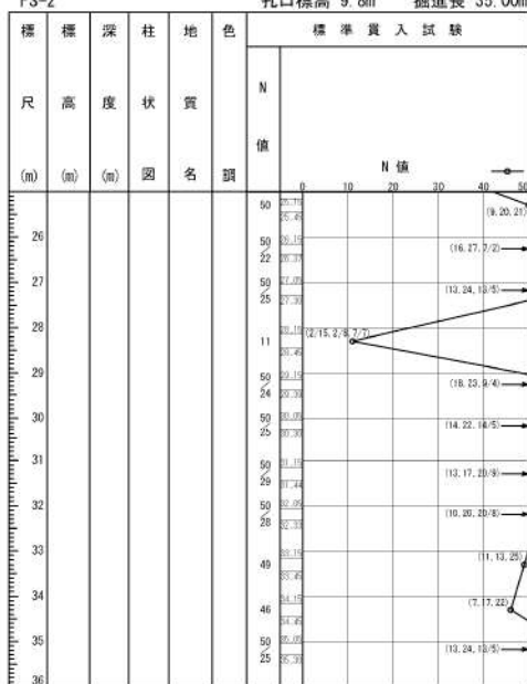
添付 1-40 図 (2/10) ボーリング柱状図・コア写真 (FS-2)
