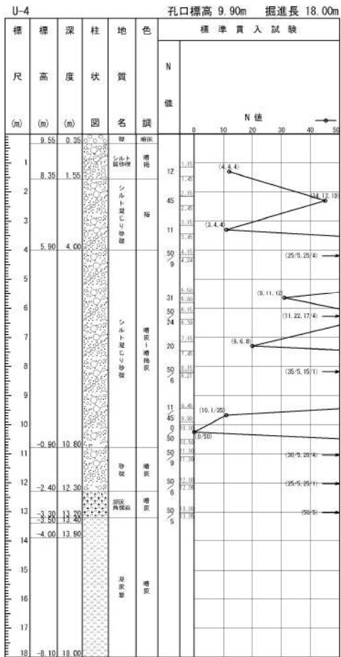
添付 1-12 図 ボーリング柱状図・コア写真 (U-4)
