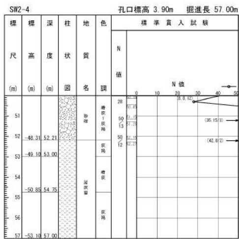
添付 1-38 図(3/3) ボーリング柱状図・コア写真 (SW2-4)
