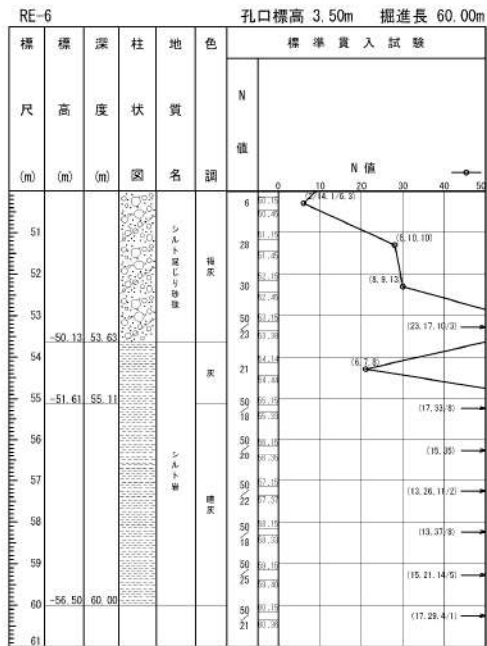
添付 1-9 図(3/3) ボーリング柱状図・コア写真 (RE-6)
