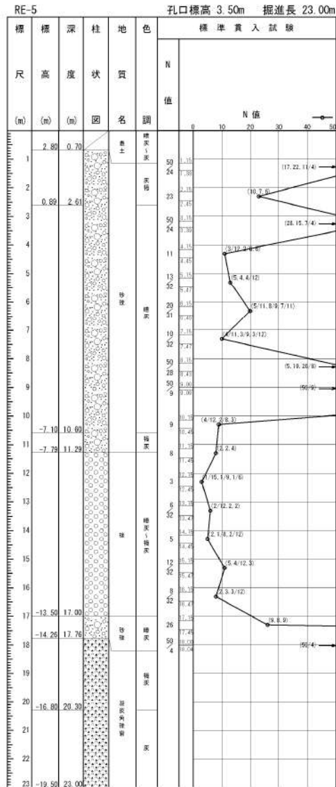
添付 1-8 図 ボーリング柱状図・コア写真 (RE-5)
