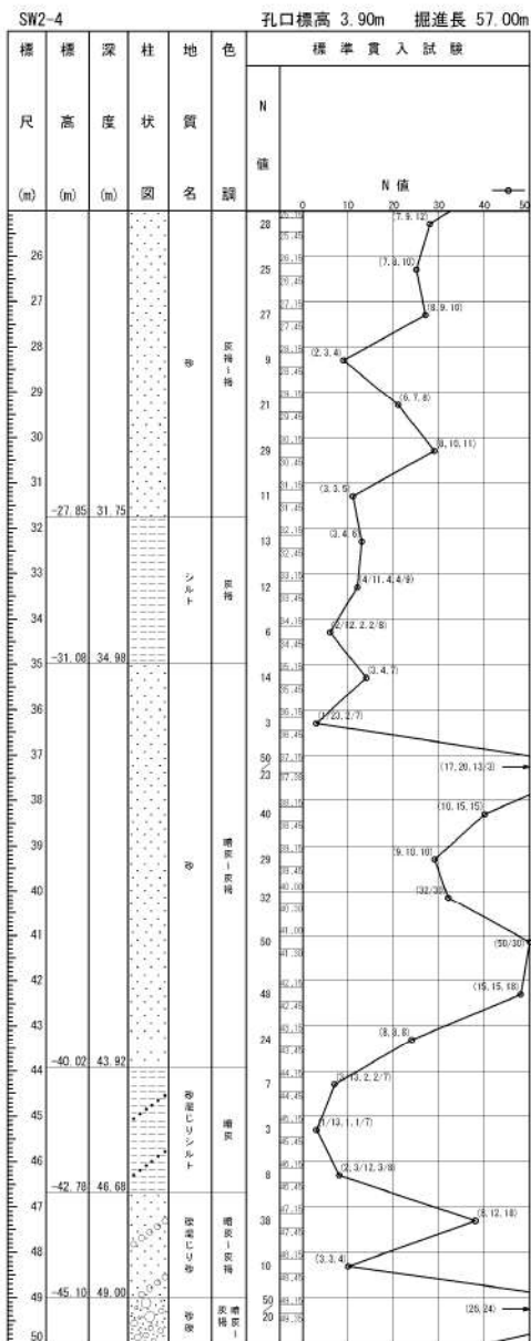
添付 1-38 図(2/3) ボーリング柱状図・コア写真 (SW2-4)
