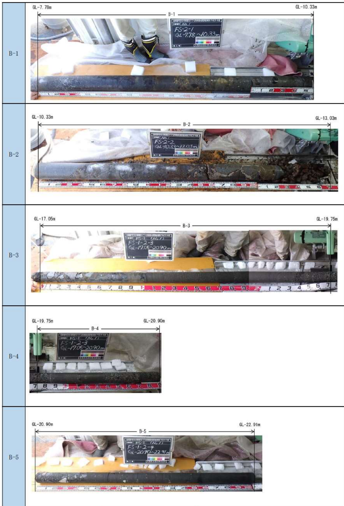
添付 1-24 図(5/10) ボーリング柱状図・コア写真 (FS-1)
