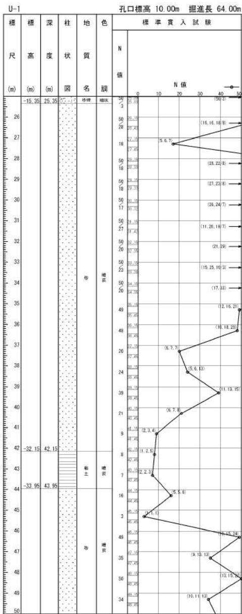
添付 1-32 図(2/3) ボーリング柱状図・コア写真 (U-1)
