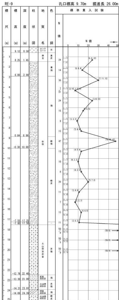
添付 1-21 図(1/2) ボーリング柱状図・コア写真 (RE-9)
