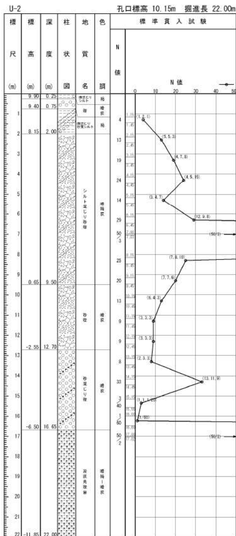
添付 1-33 図 ボーリング柱状図・コア写真 (U-2)
