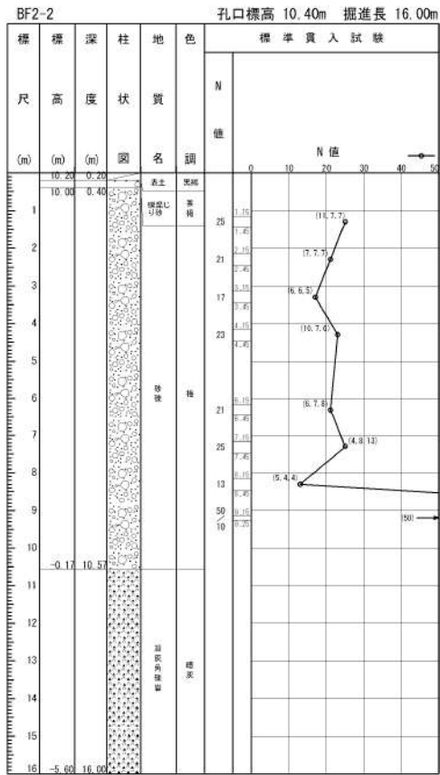
添付 1-20 図 ボーリング柱状図・コア写真 (BF2-2)
