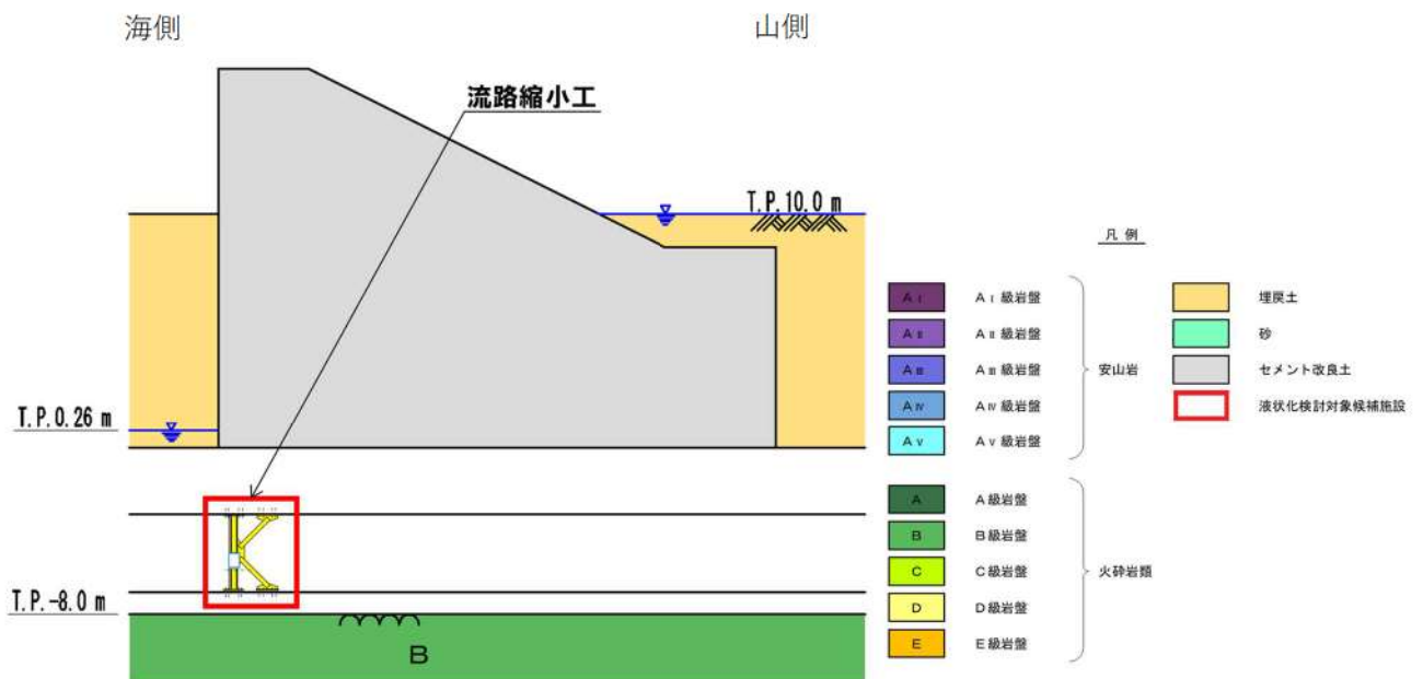
第 3.2-18 図 1 号及び 2 号炉取水路流路縮小工断面図
