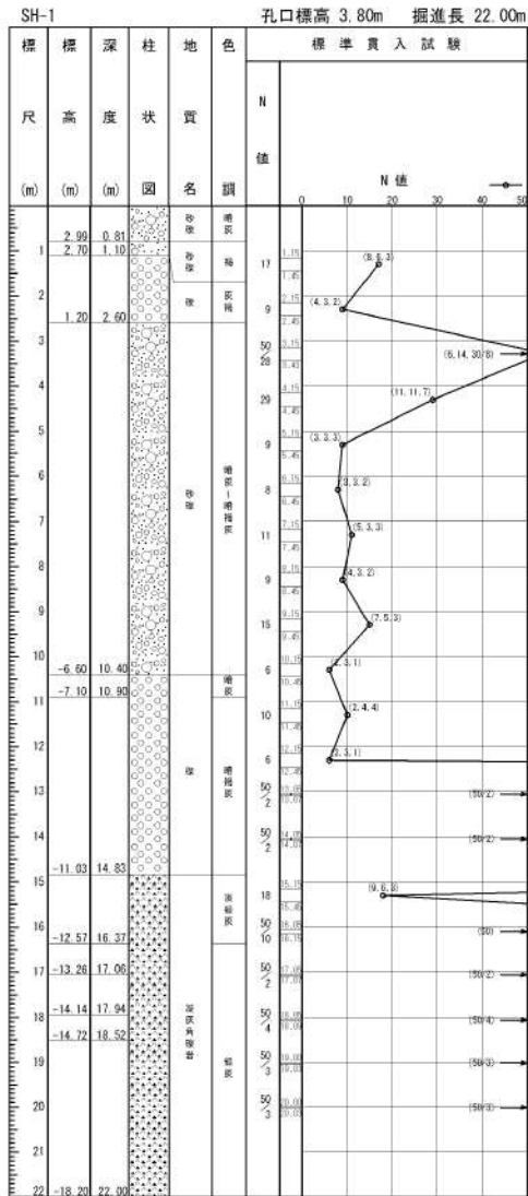
添付 1-10 図 ボーリング柱状図・コア写真 (SH-1)
