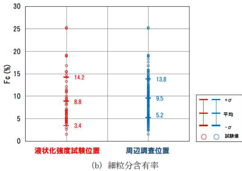
第 4.3-2 図 液状化強度試験位置の基本物性の比較(1,2号埋戻土)
