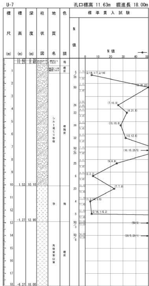
添付 1-15 図 ボーリング柱状図・コア写真 (U-7)
