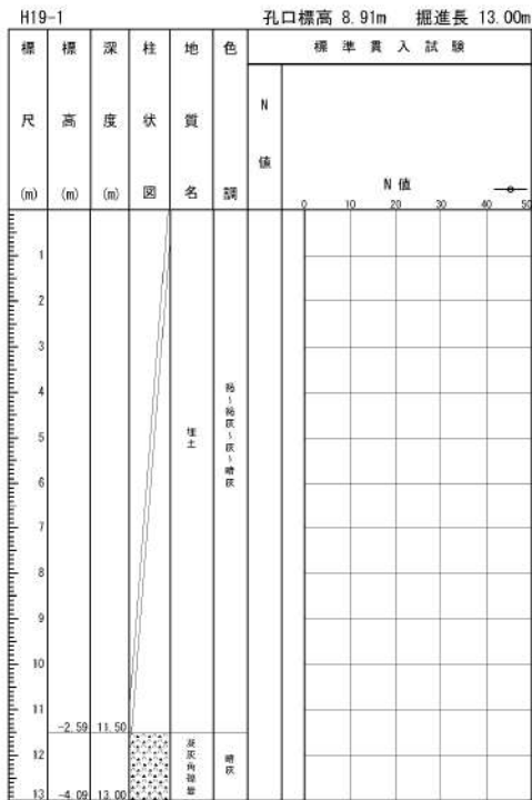
添付 1-17 図 ボーリング柱状図・コア写真 (H19-1)
