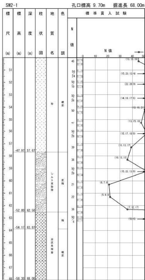
添付 1-25 図(3/3) ボーリング柱状図・コア写真 (SW2-1)
