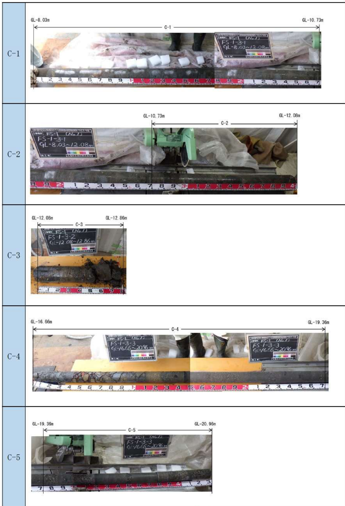
添付 1-24 図(7/10) ボーリング柱状図・コア写真 (FS-1)
