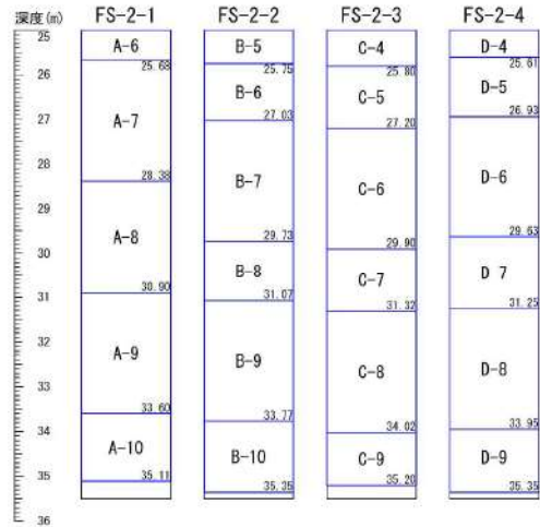
添付 1-34 図(2/10) ボーリング柱状図・コア写真 (FS-2)
