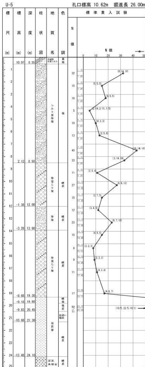
添付 1-13 図(1/2) ボーリング柱状図・コア写真 (U-5)
