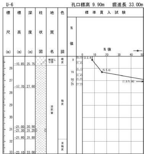
添付 1-14 図(2/2) ボーリング柱状図・コア写真 (U-6)
