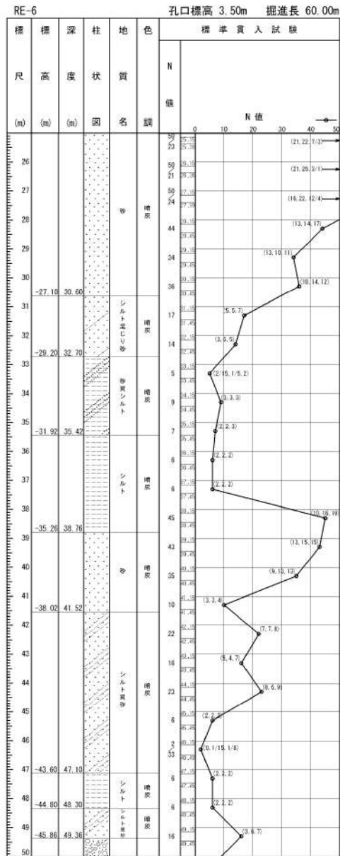
添付 1-9 図(2/3) ボーリング柱状図・コア写真 (RE-6)
