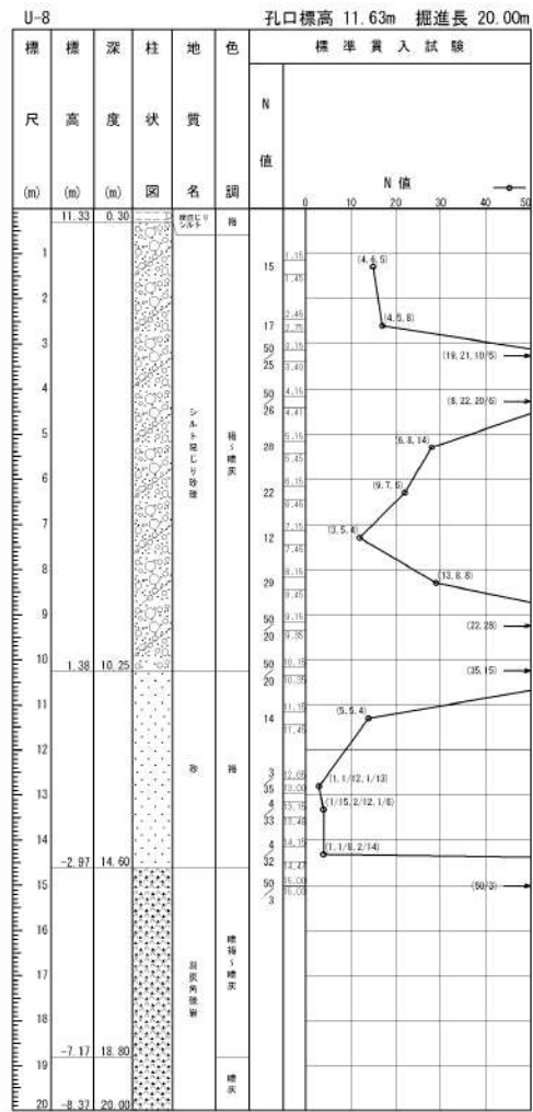
添付 1-16 図 ボーリング柱状図・コア写真 (U-8)
