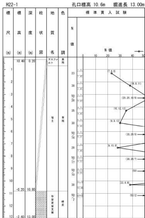
添付 1-18 図 ボーリング柱状図・コア写真 (H22-1)
