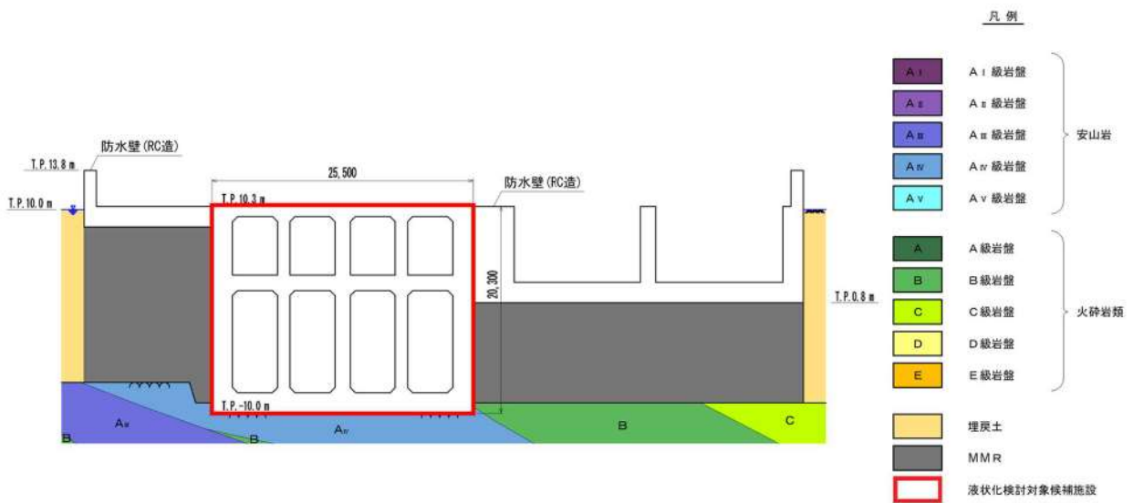
第 3.2-9 図 取水ピットスクリーン室断面図
