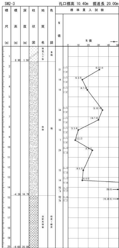
添付 1-1 図 ボーリング柱状図・コア写真 (SW2-3)
