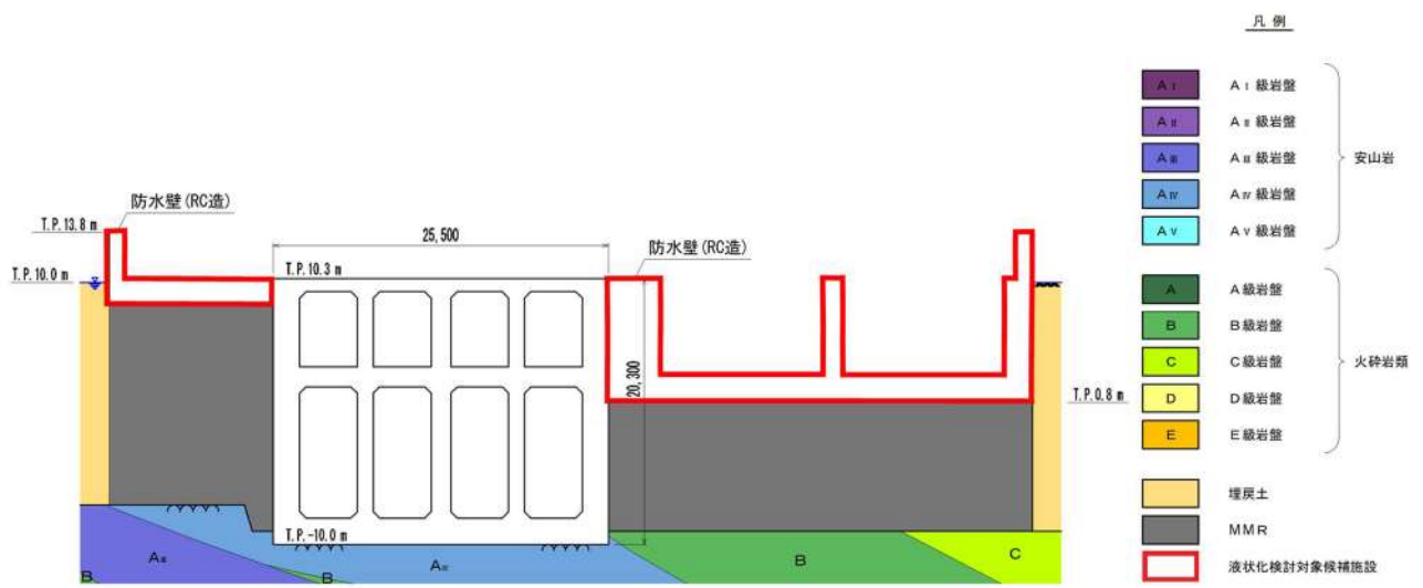
第 3.2-15 図 3号炉取水ピットスクリーン室防水壁断面図
