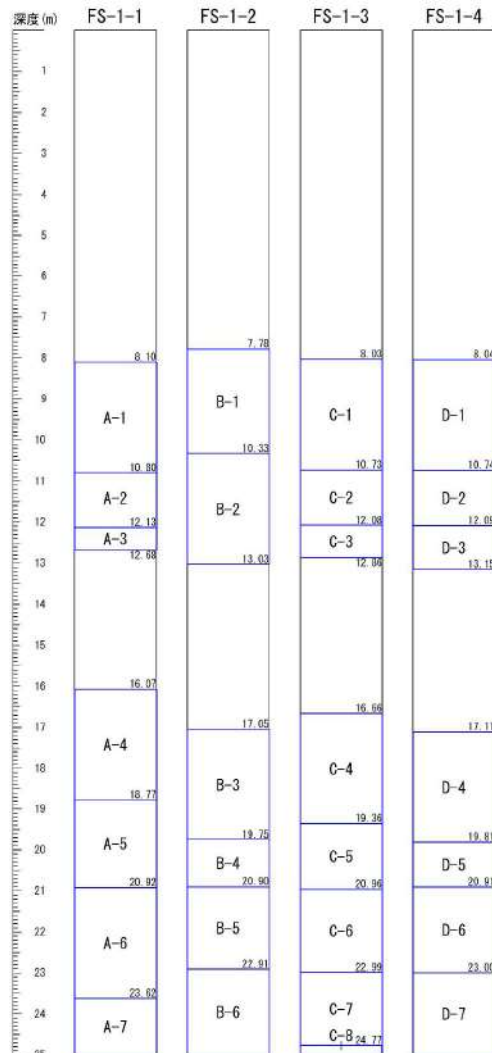
添付 1-39 図(1/10) ボーリング柱状図・コア写真 (FS-1)
