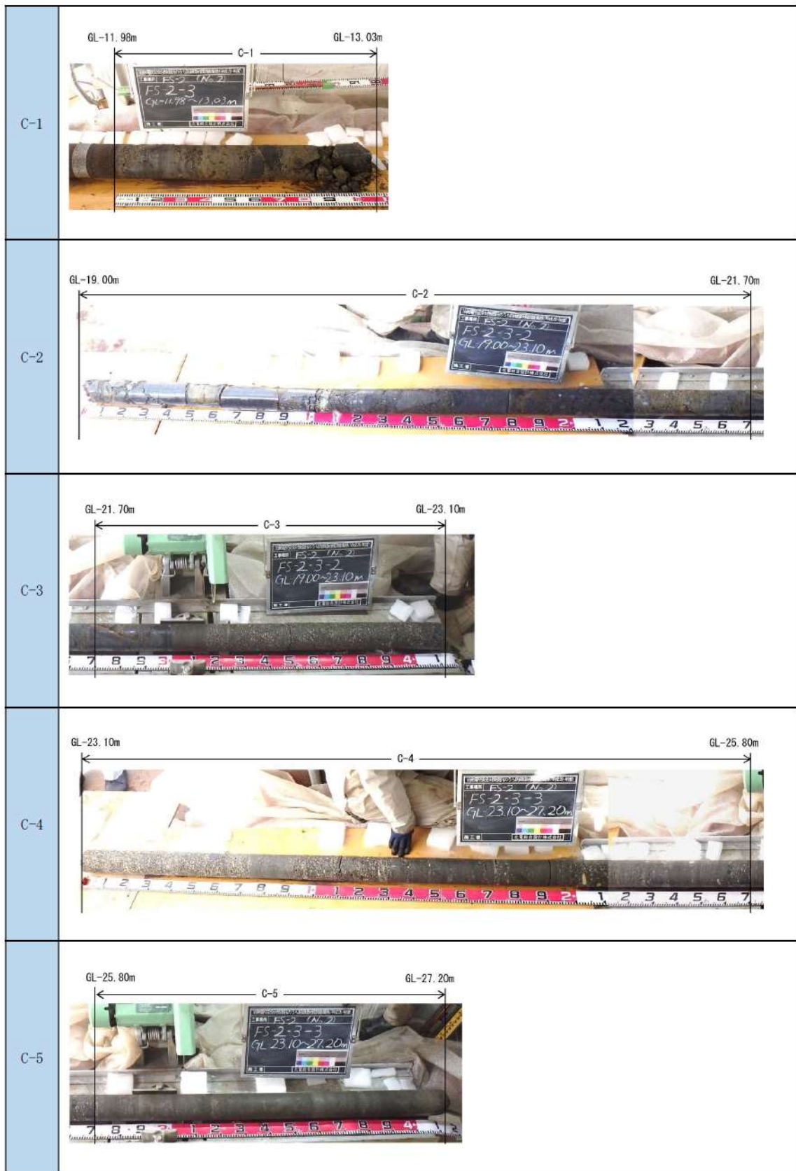
添付 1-34 図(7/10) ボーリング柱状図・コア写真 (FS-2)
