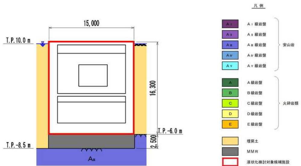
第 3.2-11 図 原子炉補機冷却海水ポンプ出口ストレーナ室断面図
