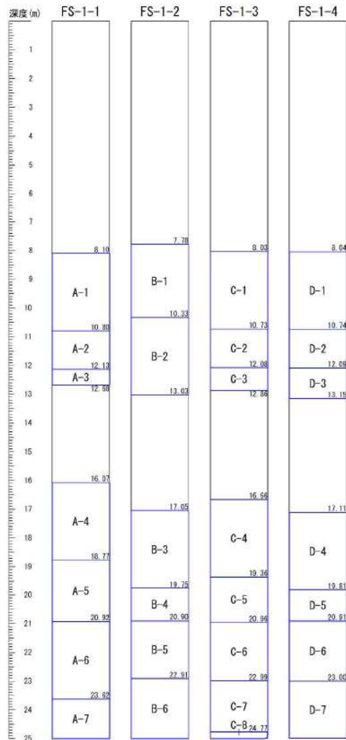
添付 1-24 図(1/10) ボーリング柱状図・コア写真 (FS-1)
