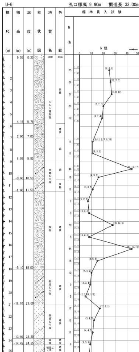
添付 1-14 図(1/2) ボーリング柱状図・コア写真 (U-6)
