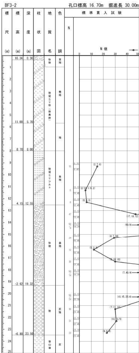
添付 1-27 図(1/2) ボーリング柱状図・コア写真 (BF3-2)
