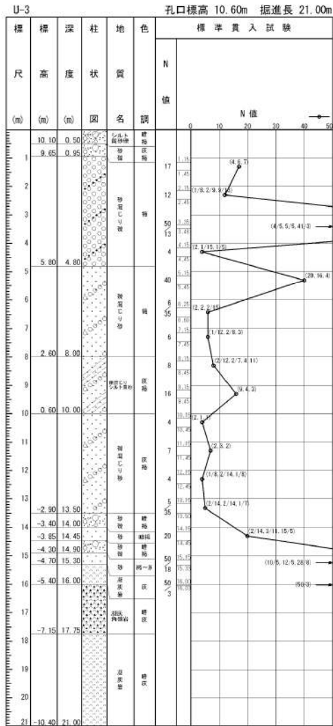
添付 1-11 図 ボーリング柱状図・コア写真 (U-3)
