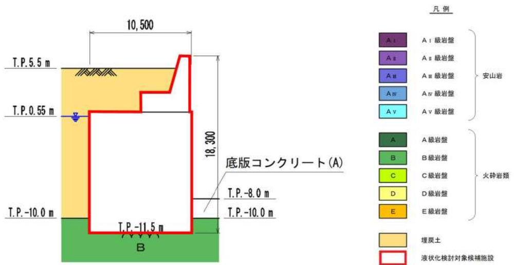
第 3.2-7 図 取水口断面図
