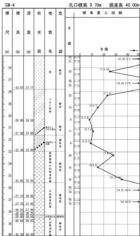
添付 1-35 図(2/2) ボーリング柱状図・コア写真 (SW-4)
