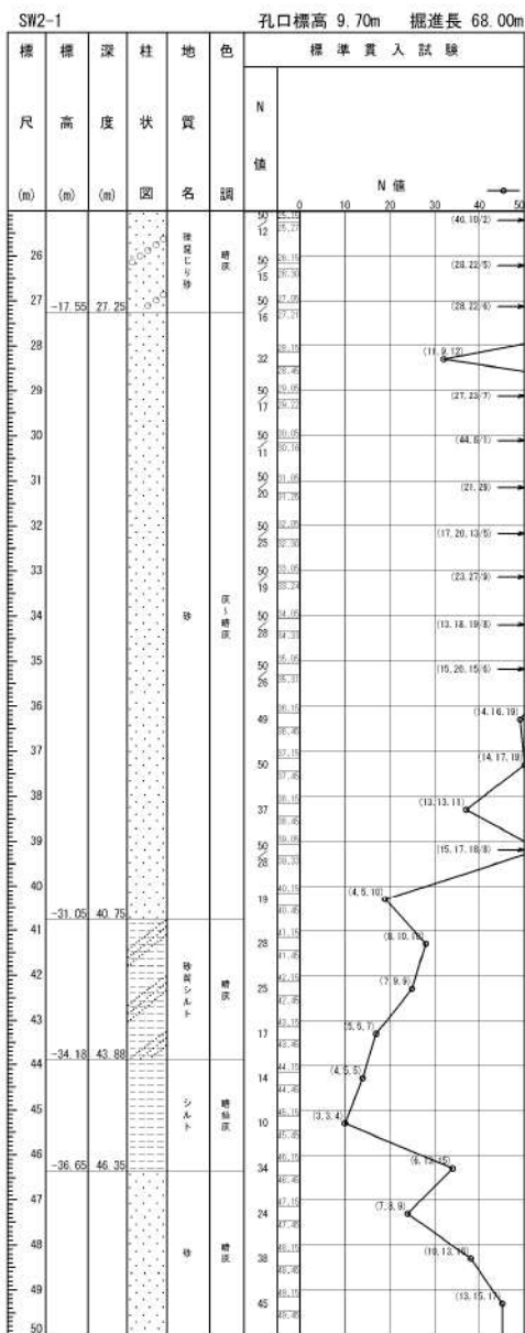
添付 1-25 図(2/3) ボーリング柱状図・コア写真 (SW2-1)
