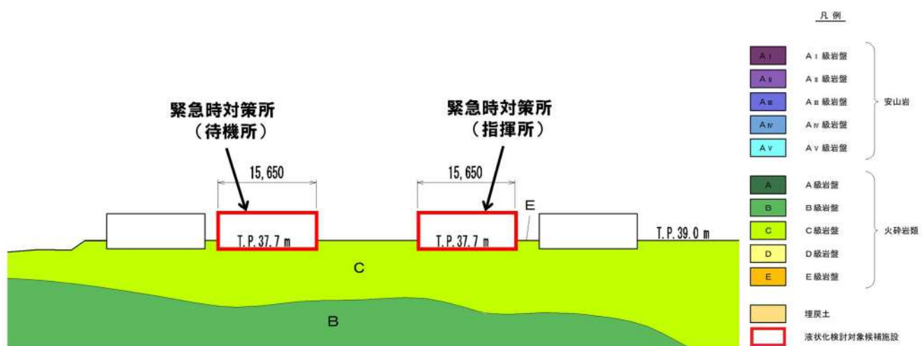
③緊急時対策所(指揮所, 待機所)断面図(③-③')
