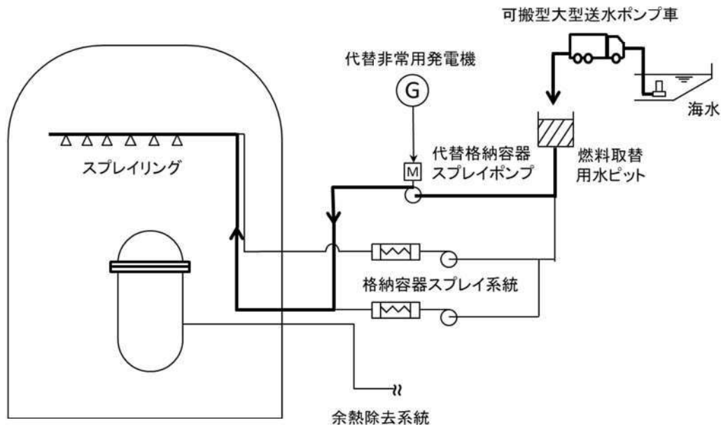
図 1 概略系統図
