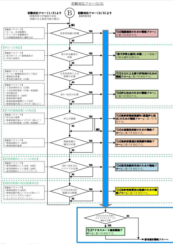
第2図 初動対応フロー (3/3)
