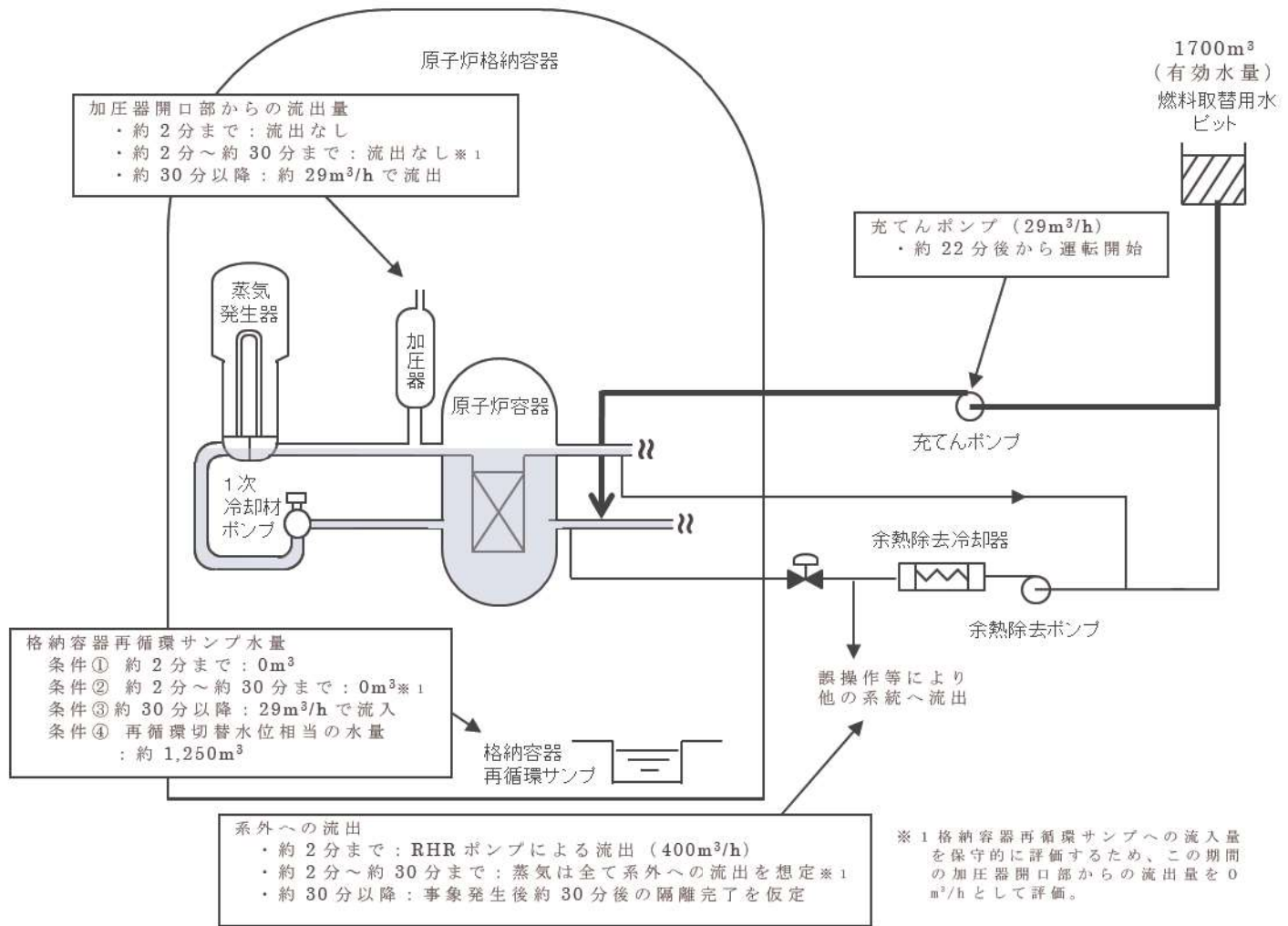
図 1 再循環切替水位に到達するまでの時間評価の想定 (ミッドループ運転中の原子炉冷却材の流出)
