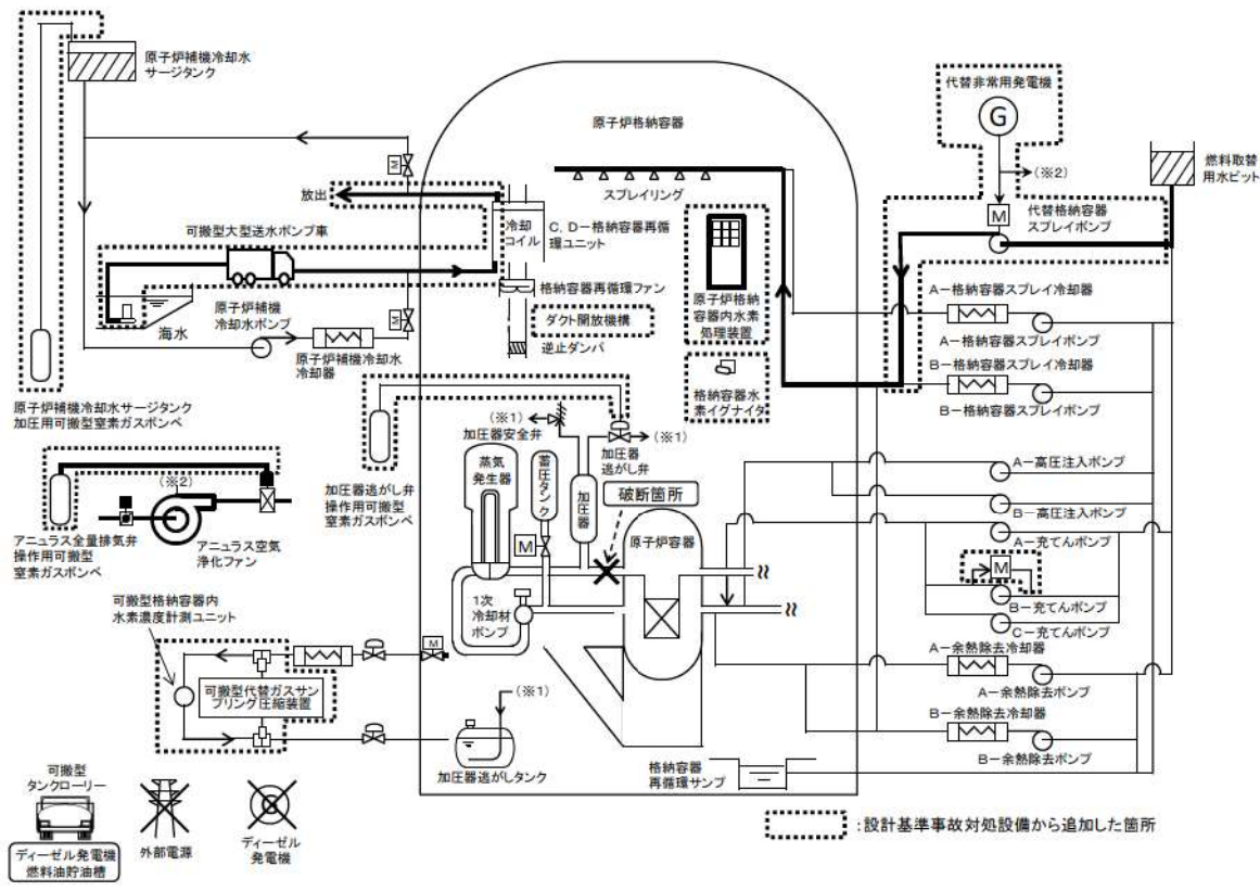
第 7.2.4.1 図 「水素燃焼」の重大事故等対策の概略系統図 (原子炉格納容器内水素処理装置及び格納容器水素イグナイタ)
