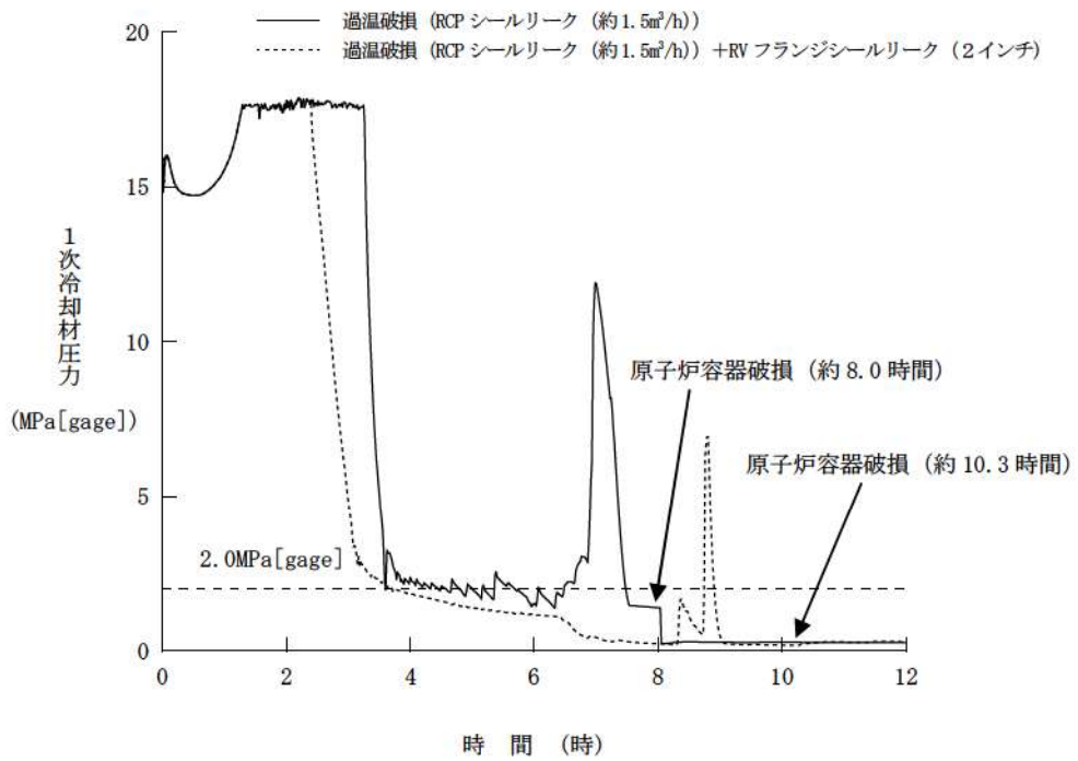
図 3-4 1次冷却材圧力
