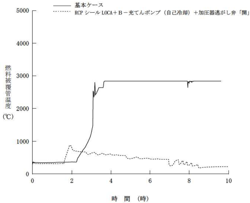
図 3-3 燃料被覆管温度
