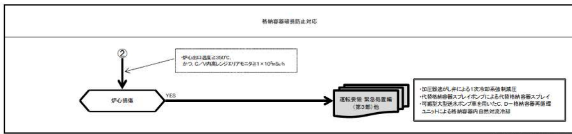
第 7.2.1.2.4 図 「雰囲気圧力・温度による静的負荷（格納容器過温破損）」の事象進展（判定プロセス） （外部電源喪失時に非常用所内交流電源が喪失し、補助給水機能が喪失する事故）（2 / 2）
