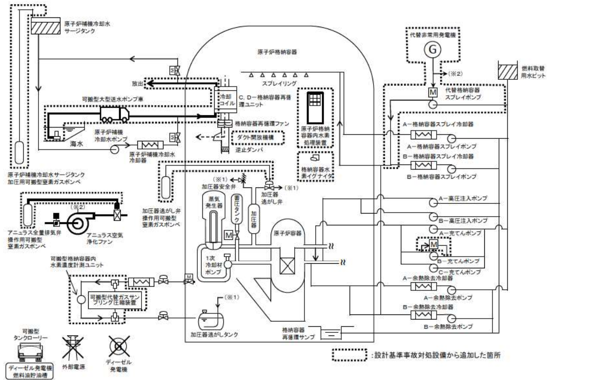
第 7.2.1.2.1 図 「雰囲気圧力・温度による静的負荷（格納容器過温破損）」
