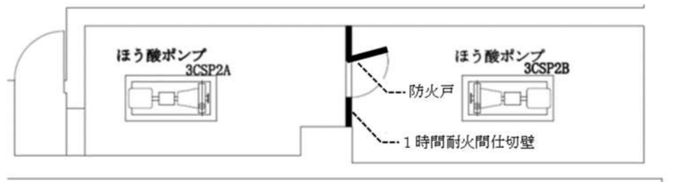
第9図：隔壁設置箇所の火災区画平面図
