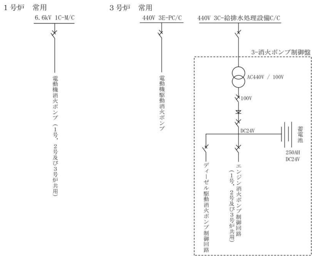
第 1-17 図：消火設備の電源確保の概要
