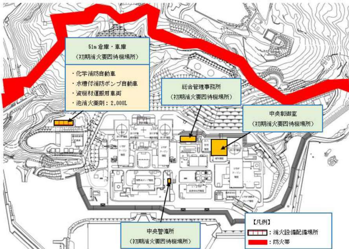
第 1-16 図：移動式消火設備の配置の概要
