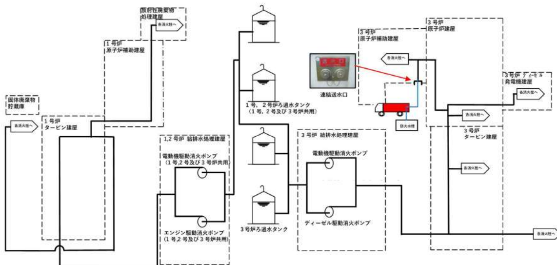
第 1-22 図：給水接続口接続概要図
