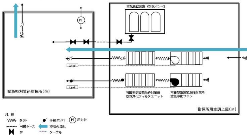
第1.18.19図 可搬型空気浄化装置運転概要図
