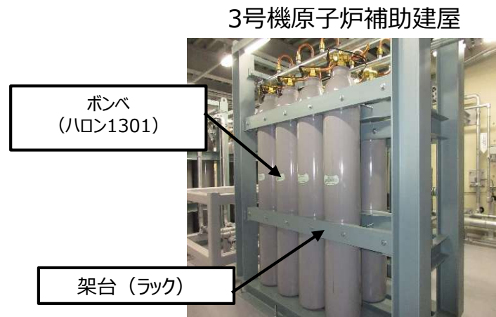
図17 発電所におけるボンベの設置状況
