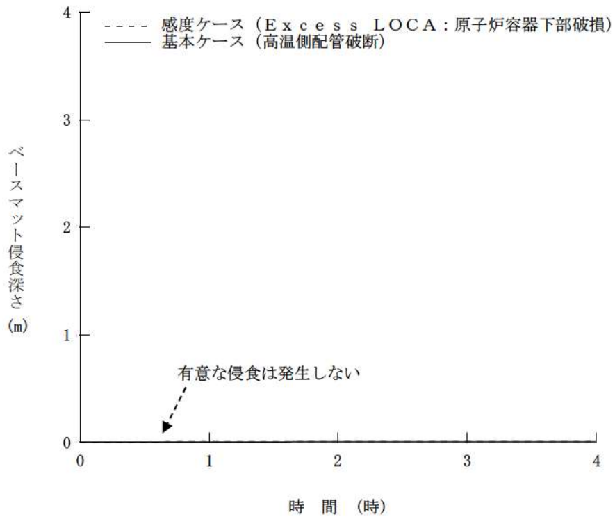
図 15 ベースマツト侵食深さ (壁面) の推移 (原子炉容器下端における破損時の影響確認)
