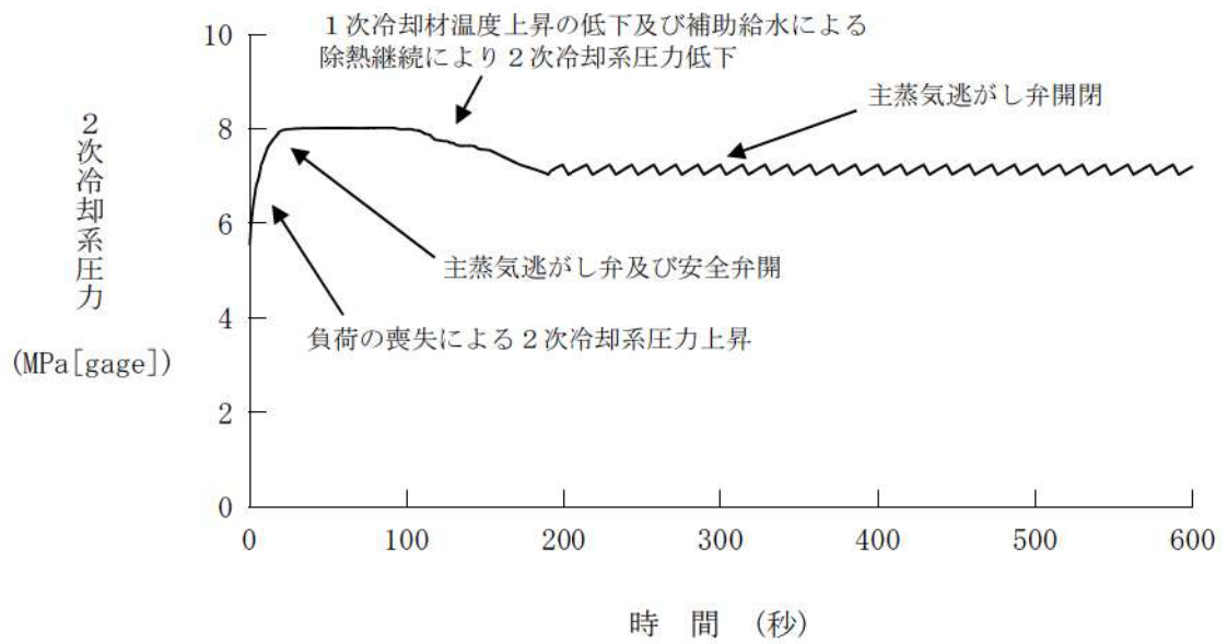
第7.1.5.27図 2次冷却系圧力の推移（負荷の喪失）
