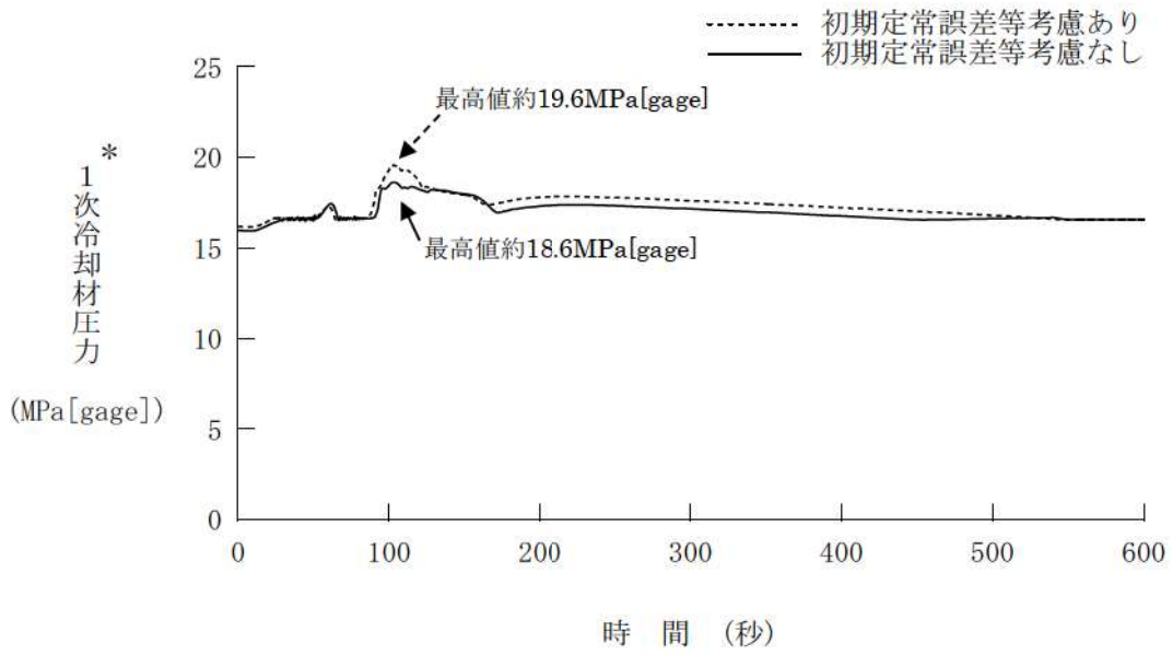
第 7. 1. 5. 30 図 1次冷却材圧力の推移比較（主給水流量喪失） （初期定常誤差及びドップラ効果の感度確認）
