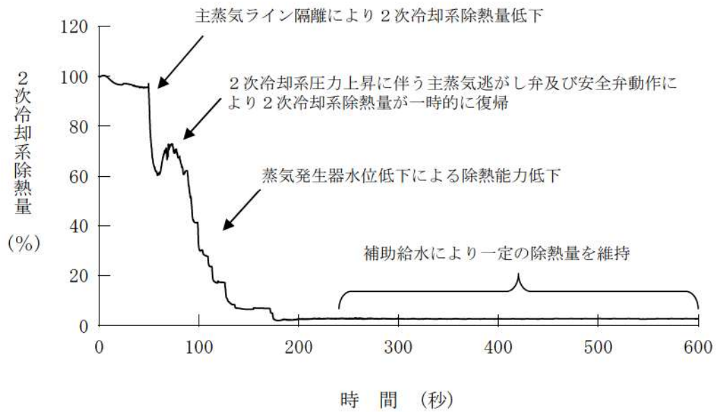
第 7. 1. 5. 13 図 2 次冷却系除熱量の推移 (主給水流量喪失)
