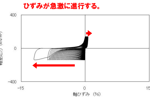
③④ 軸差応力-軸ひずみ関係
