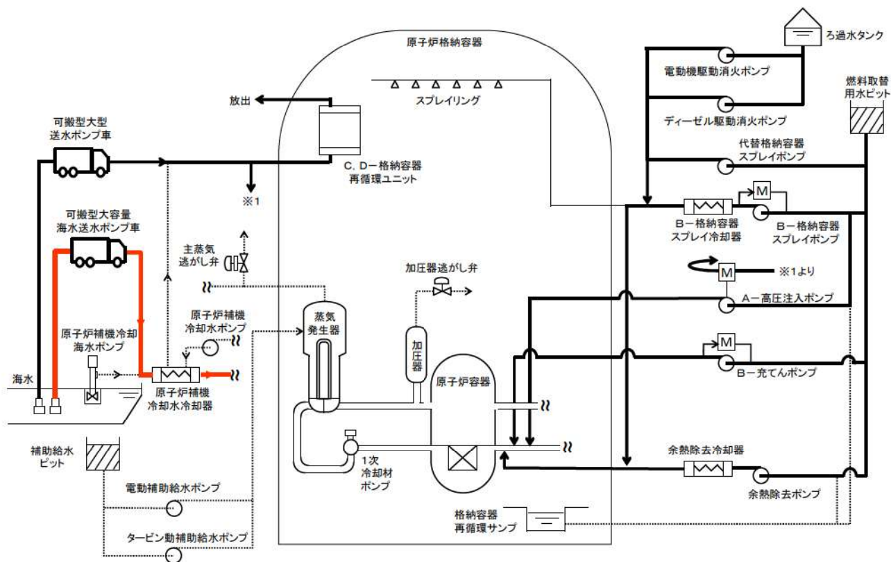
図2 概略系統図
