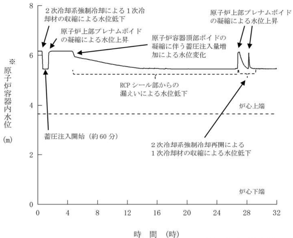
第 7.1.2.34 図 原子炉容器内水位の推移 (RCP シール LOCA が発生しない場合)
