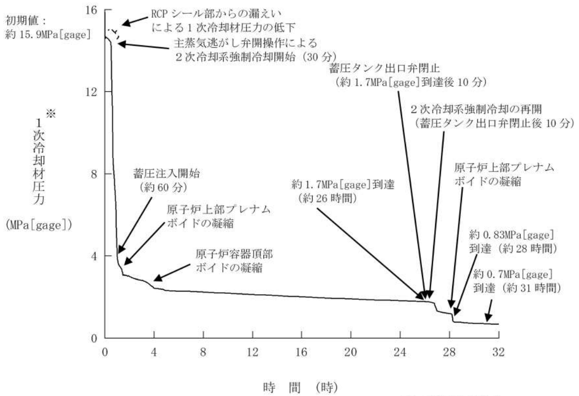
第 7.1.2.27 図 1次冷却材圧力の推移 (RCP シール LOCA が発生しない場合)
