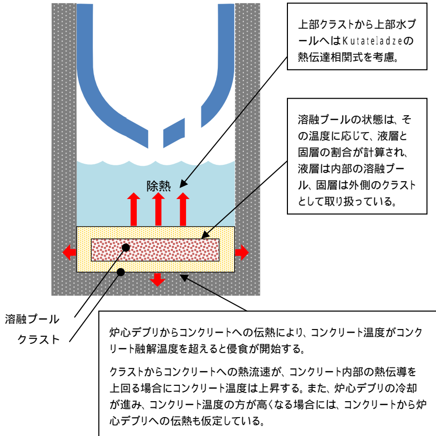
図 4-1 炉心デブリ伝熱の想定される現象と解析上の取り扱いとの比較概念図 (2/2)
