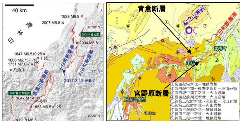
長野県北部の主な地震
