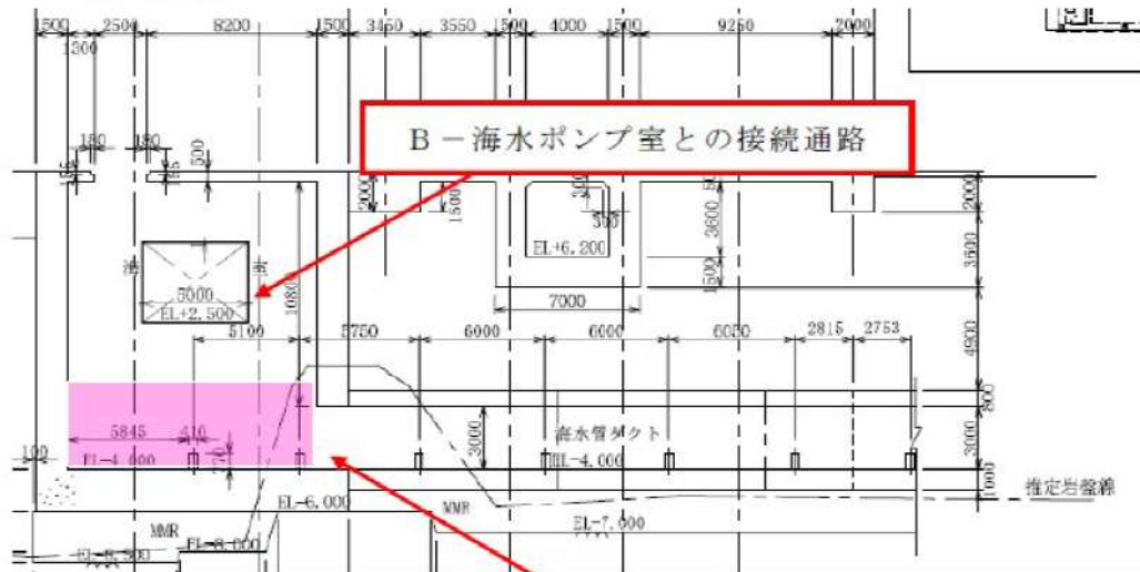
【断面図】
