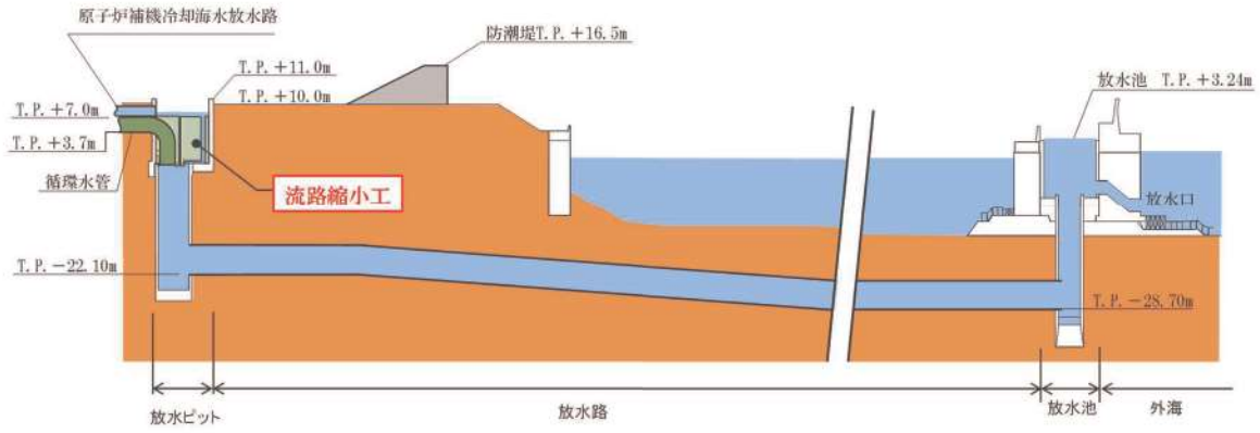
第 1.5. ● 図 3号炉放水系統断面図
