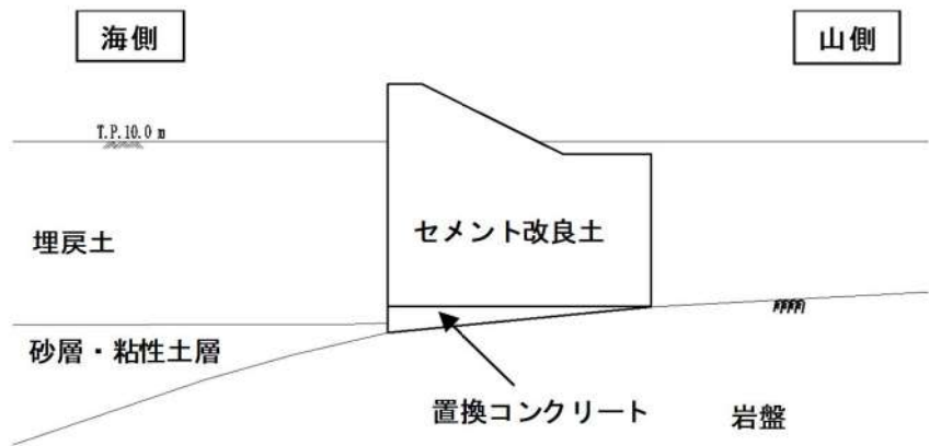
防潮堤 断面図
