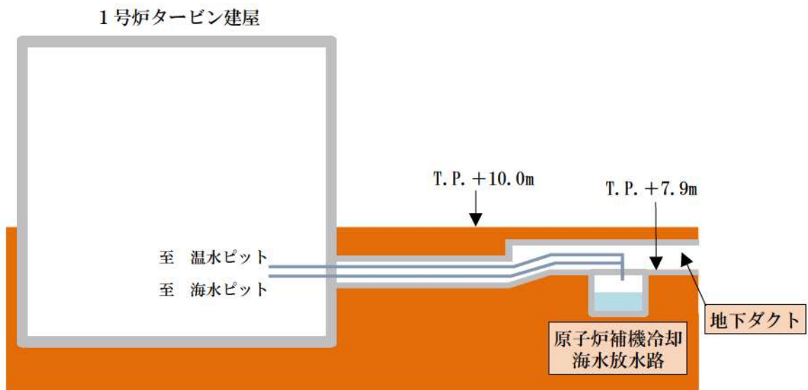
図 2.2-22 温水ピット及び海水ピット排水ライン 概要図 (A-A 断面)
