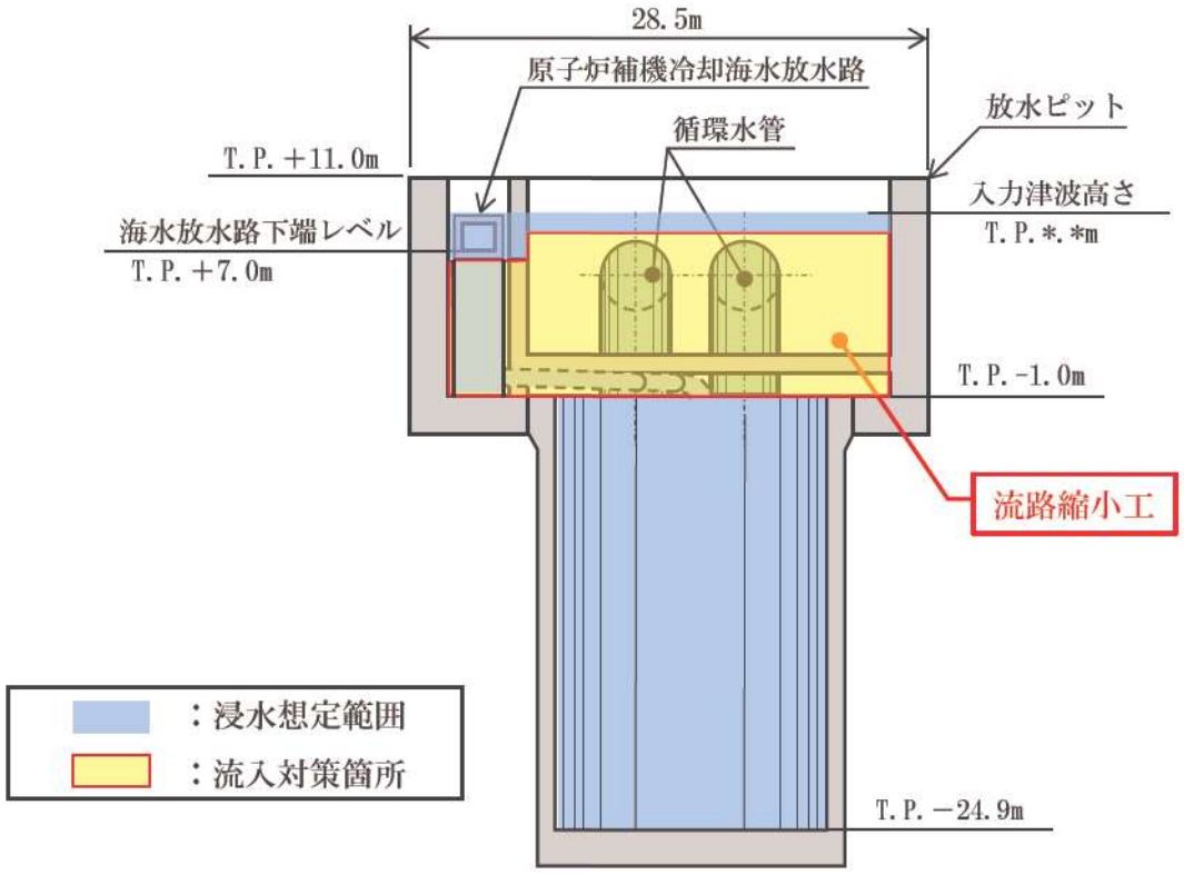
第 10.6. ● 図 流路縮小工概念図
