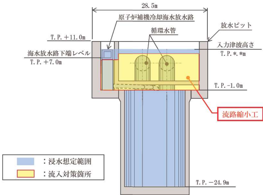
第 1.5. ● 図 3号炉放水ピット断面図
