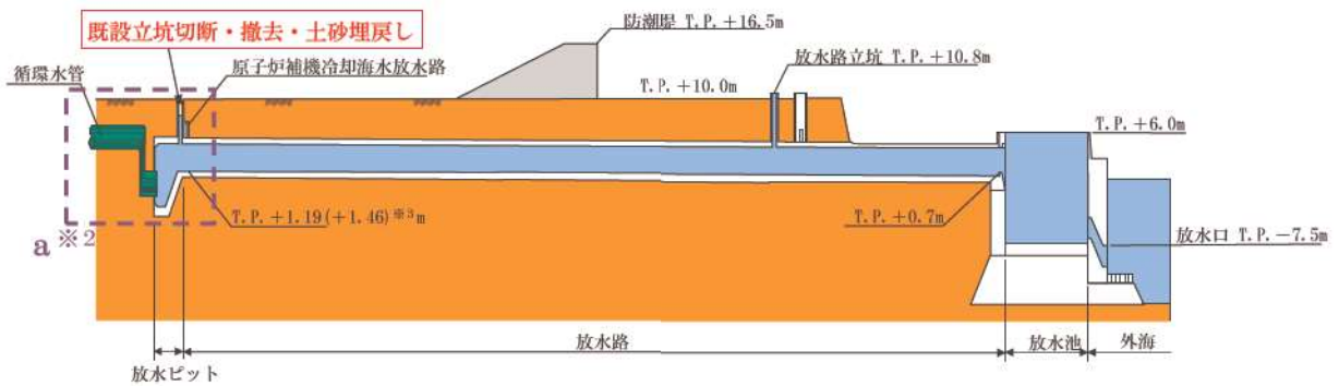
【A-A 断面】
