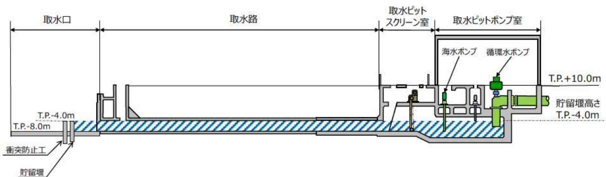
第 10.8. ●図 非常用取水設備概要図
