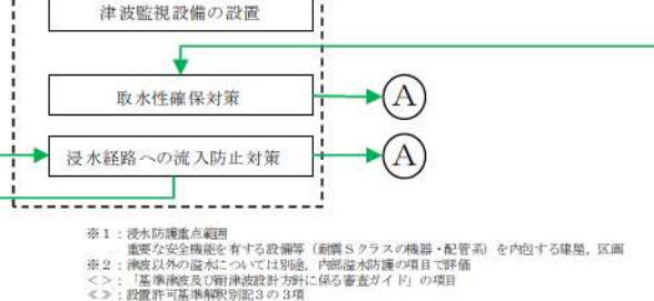
図1 津波による損傷防止の確認フロー
