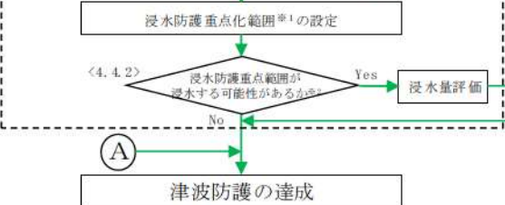
図1 津波による損傷防止の確認フロー
