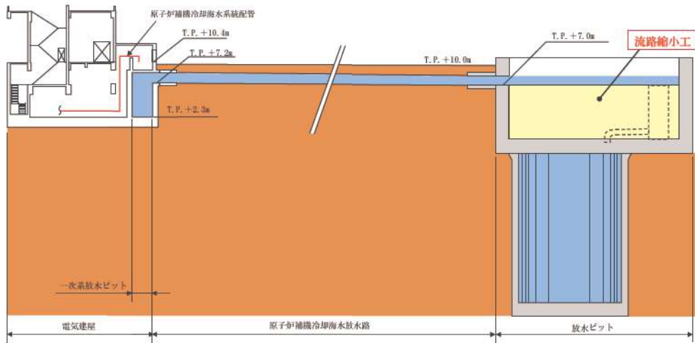
【B-B 断面】
