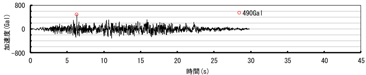
乱数位相波__加速度時刻歴波形(鉛直方向)
