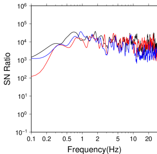
2014/7/8胆振地方の地震(M5.6) IBUH07大滝
