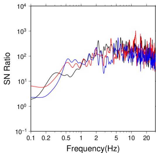
2017/8/13後志地方の地震(M3.5) SBSH04共和
