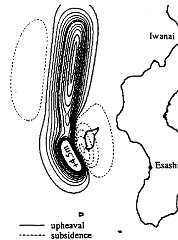
図1 地盤変位
