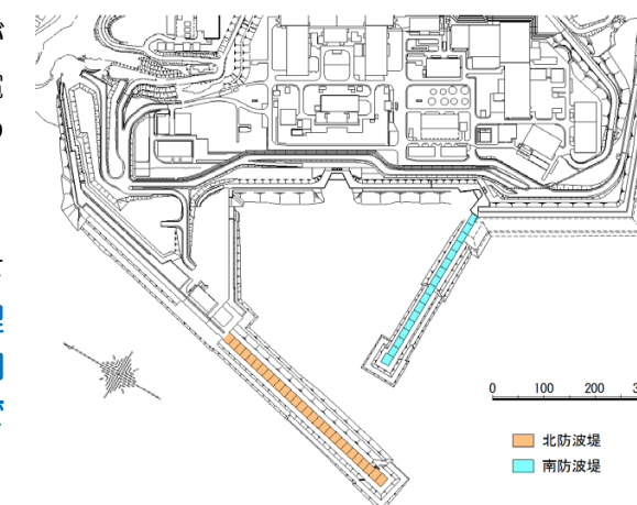
泊発電所防波堤配置図
