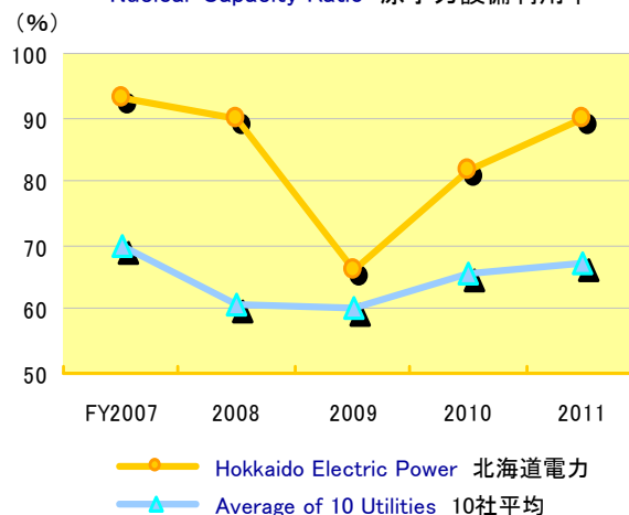
Nuclear Capacity Ratio 原子力設備利用率
